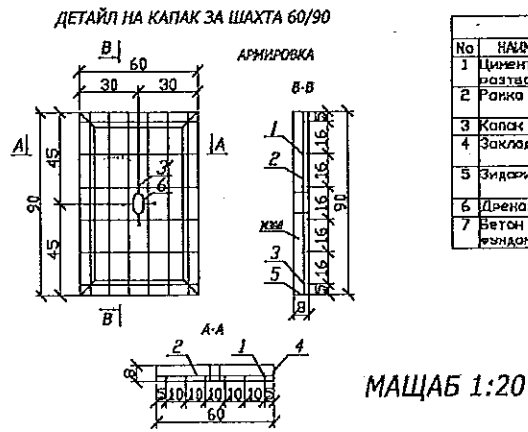
Фиг.6.3. Кабелна шахта – единична
